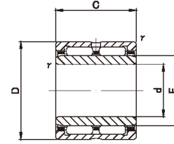
NA69
