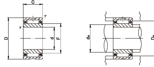
NA49,NA59,NA69(d ≤ 30),NK
