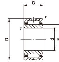
NA49,NA59,NA69(d ≤ 30),NKI
