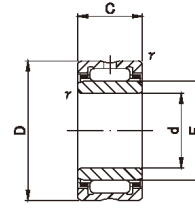
NA49,NA59,NKI
