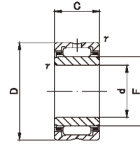
NA49,NA59,NA48,NKI
