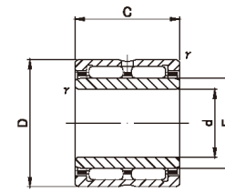
NA69
