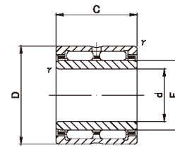
NA69
